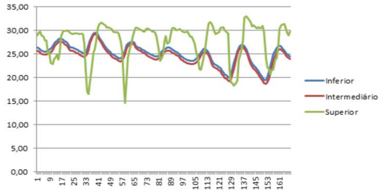
Figura 9. Comportamento das temperaturas internas do biodigestor durante à terceira semana
