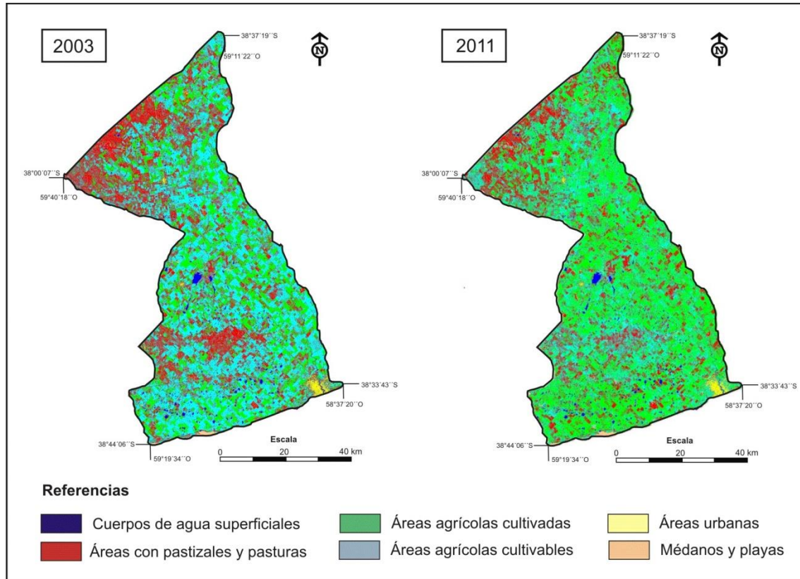
Figura 02 - Clasificación supervisada de imágenes LANDSAT 5.
