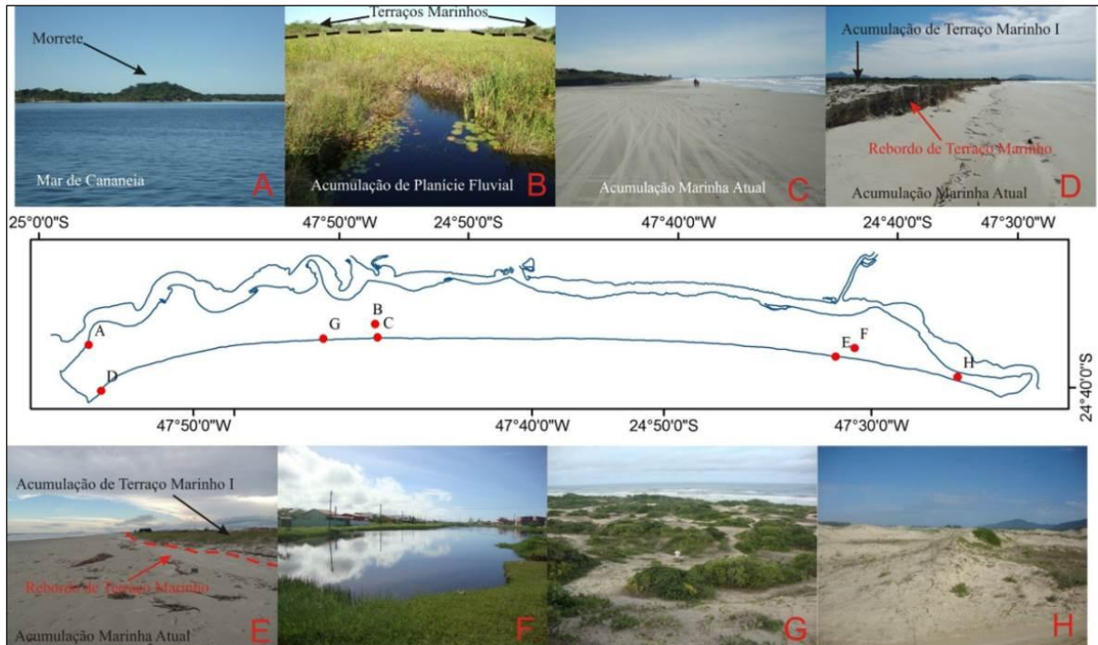
Figura 3– Compartimentos e formas de relevo da Ilha Comprida.
