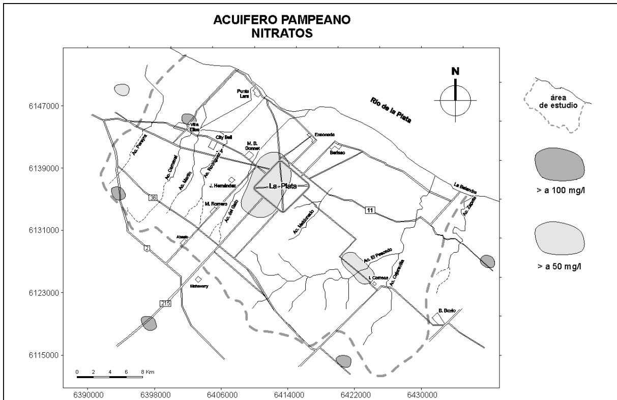
Figura 12 – Acuífero Pampeano: Nitratos
