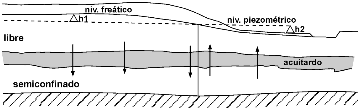
Figura 3 - Potenciales hidráulicos naturales - acuífero libre y semiconfinado
