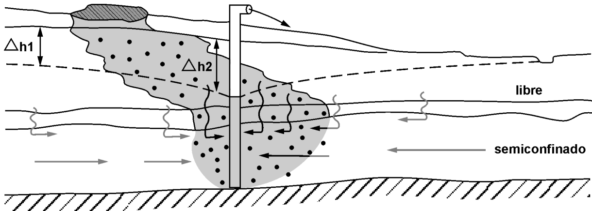
Figura 4 - Contaminación por bombeo - acuífero semiconfinado
