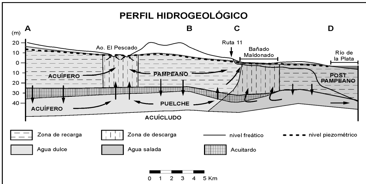
Figura 8 – Perfil Hidrogeológico
