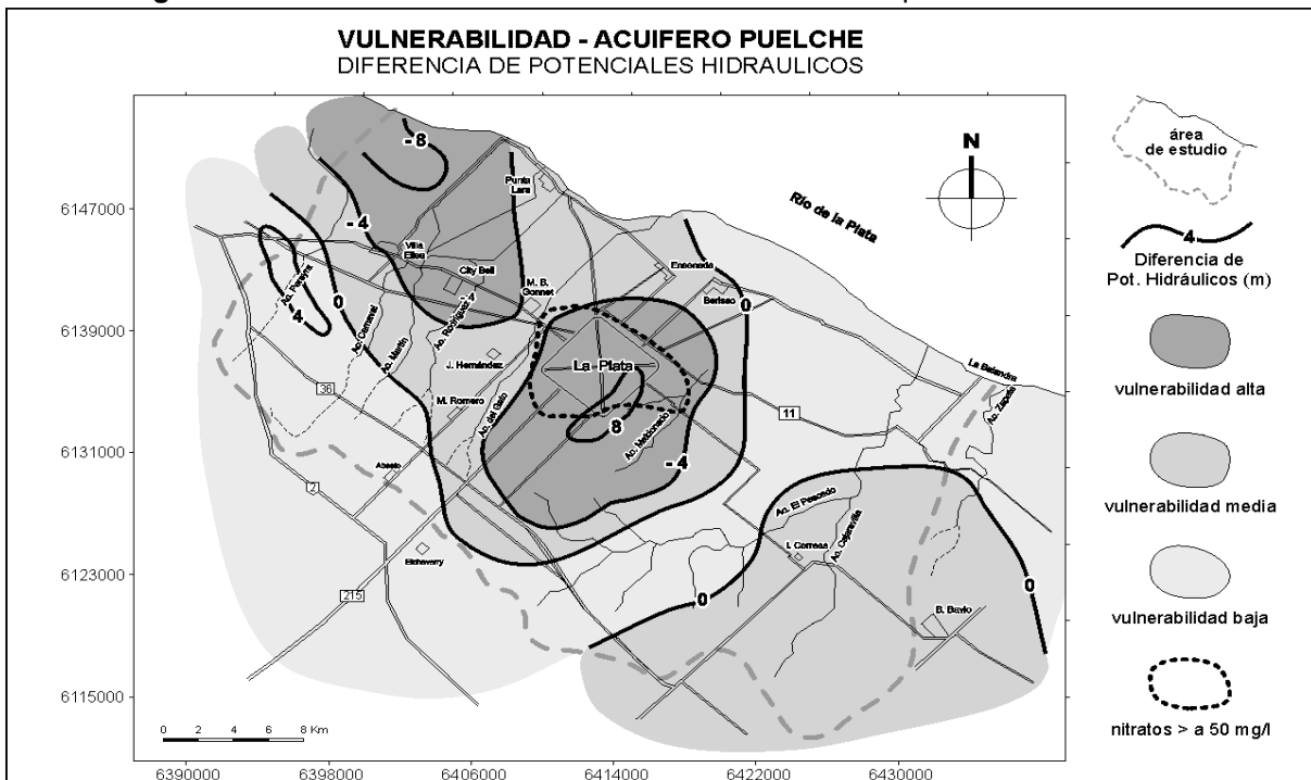
Figura 14 - Vulnerabilidad - Acuífero Puelche: diferencia de potenciales hidráulicos
