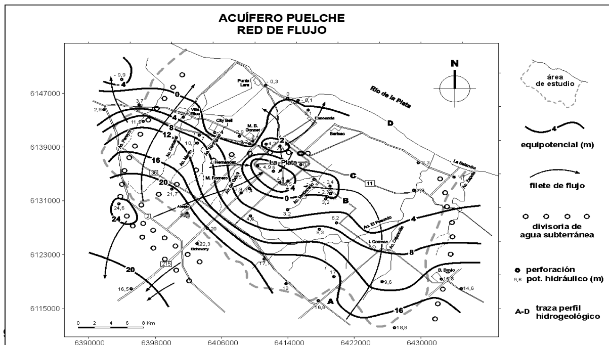
Figura 9 – Acuífero Puelche: Red de Flujo
