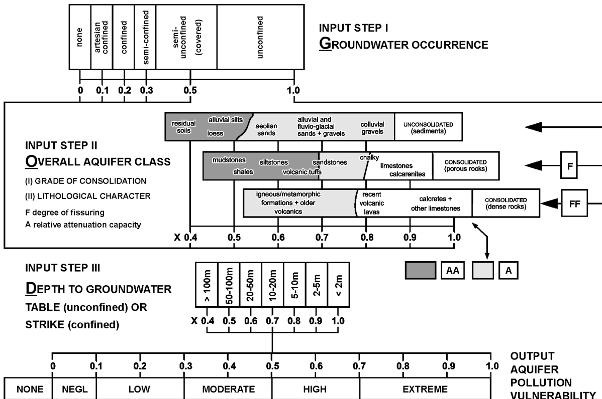
Figura 2 – Vulnerabilidad de un acuífero a la contaminación
