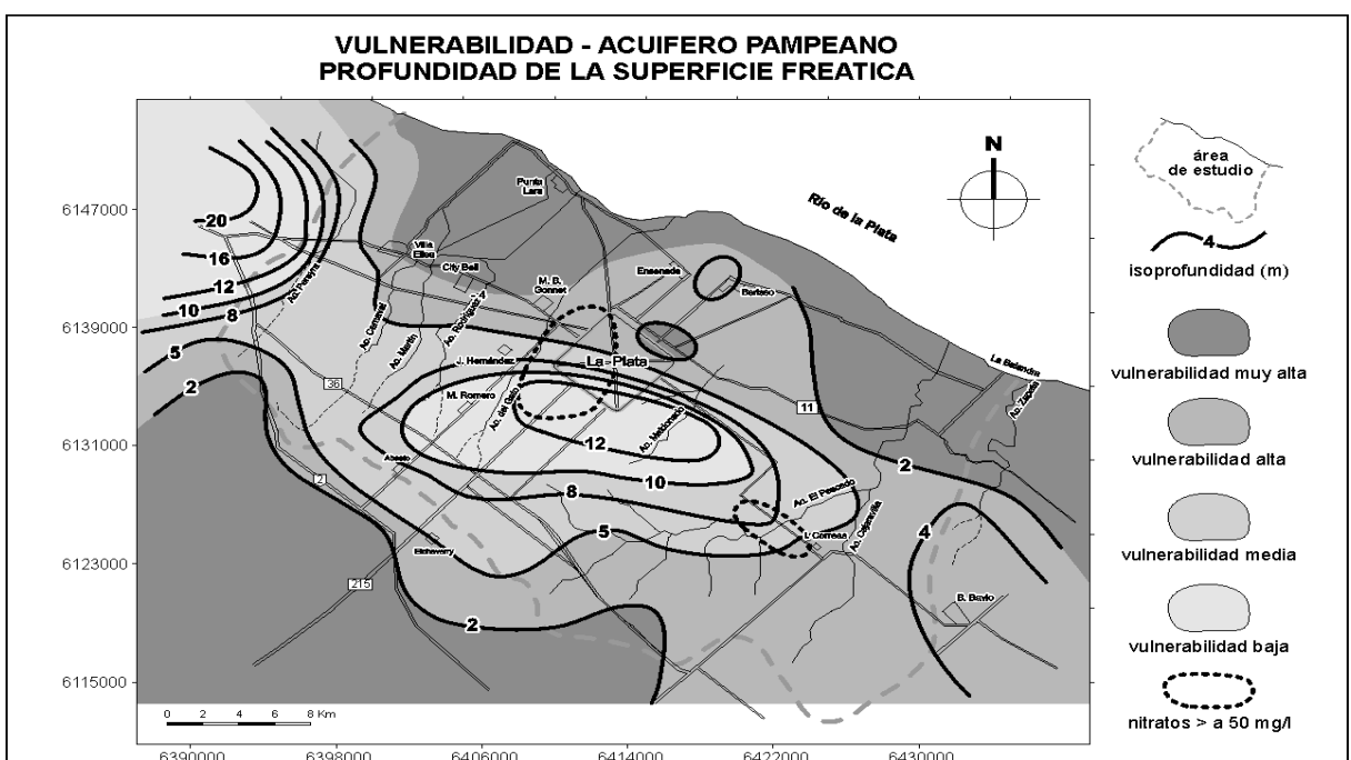
Figura 16 - Vulnerabilidad - Acuífero Pampeano: profundidad de la superficie freática
