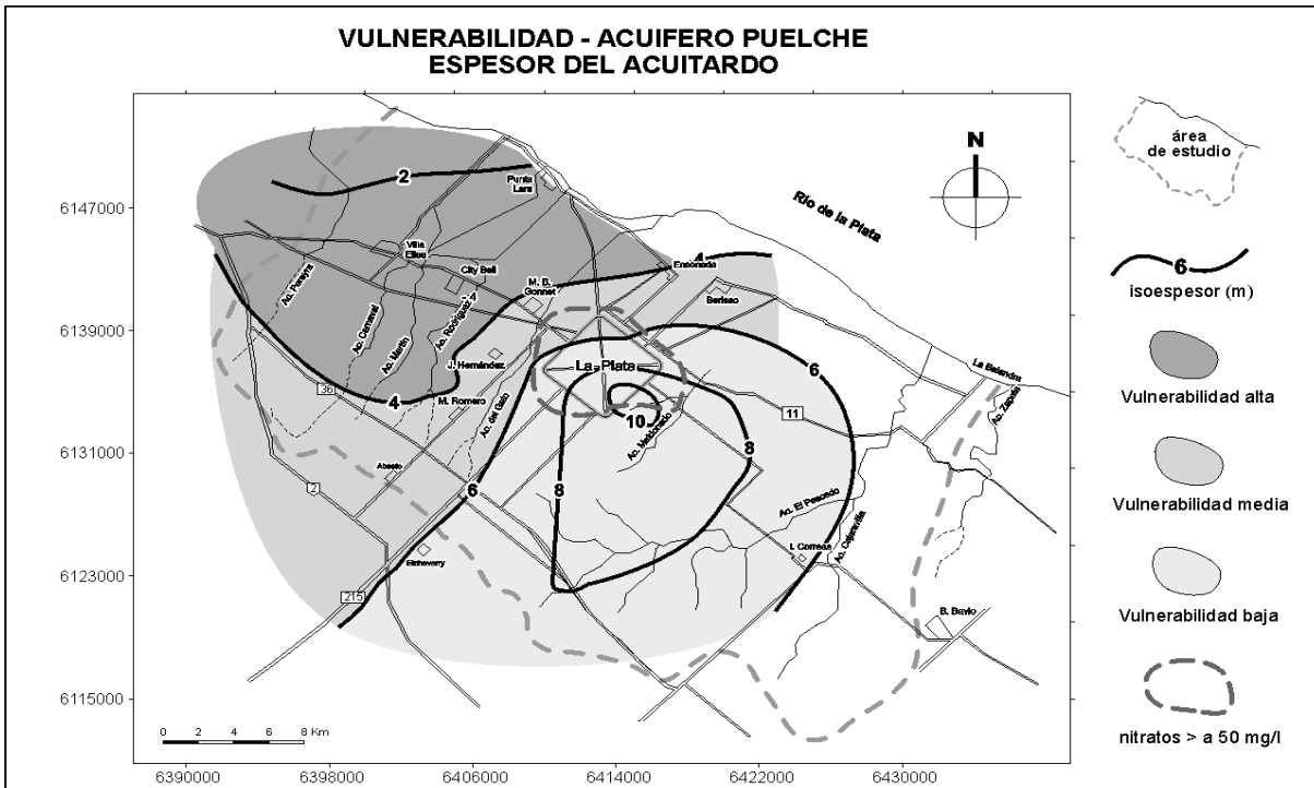
Figura 13 – Vulnerabilidad - Acuífero Puelche: espesor del acuitardo
