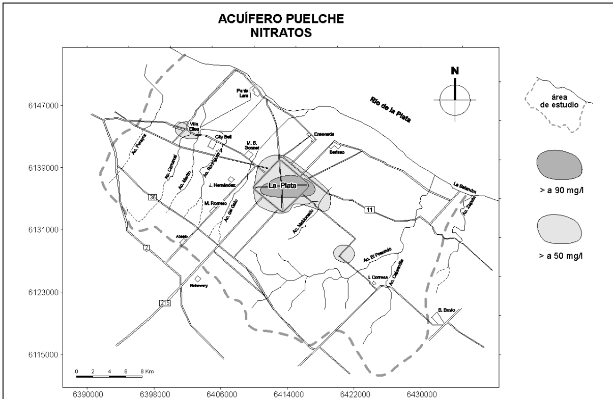
Figura 11 – Acuífero Puelche: Nitratos
