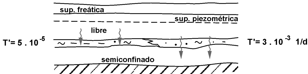
Figura 7 - Flujo a través del acuitardo por variación de la transmisividad vertical
