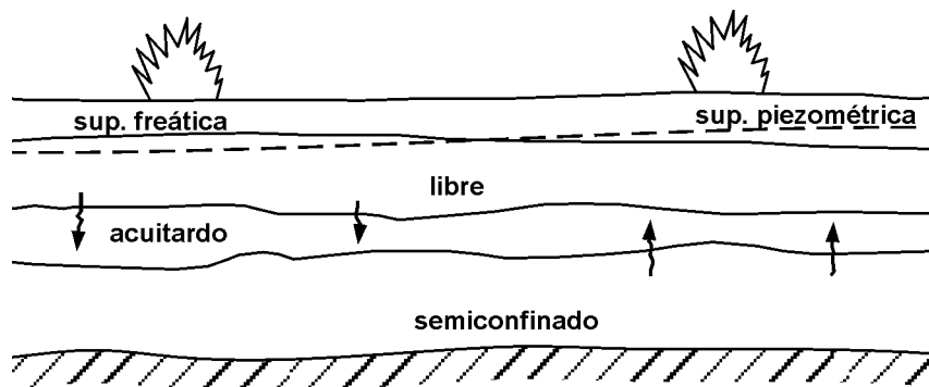
Figura 5 - Flujo a través del acuitardo - potenciales hidráulicos naturales
