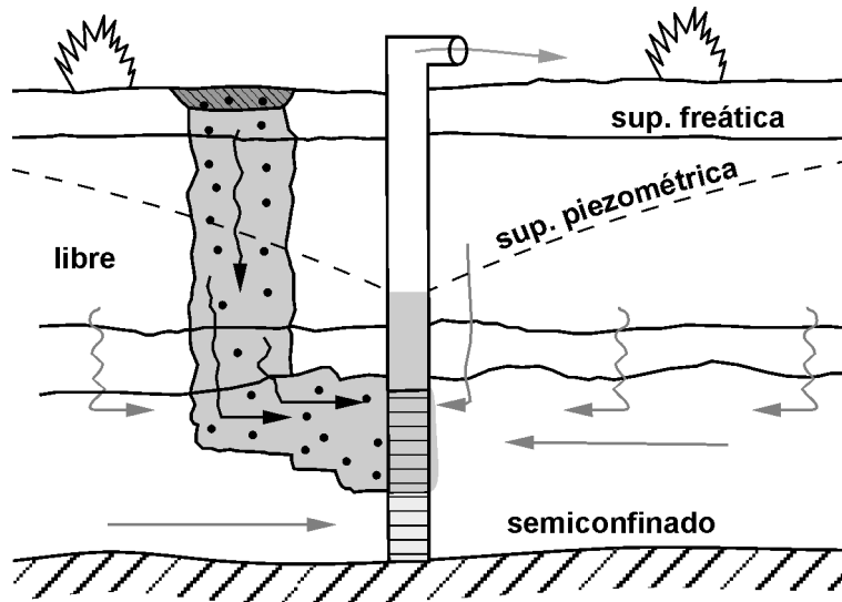
Figura 6 - Flujo a través del acuitardo - potenciales hidráulicos artificiales
