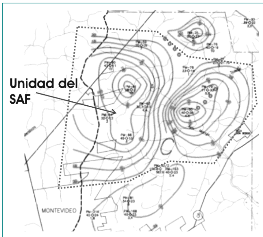
Figura 3. Unidad del SAF - Mapa potenciométrico Cuenca A° Carrasco, Uruguay
