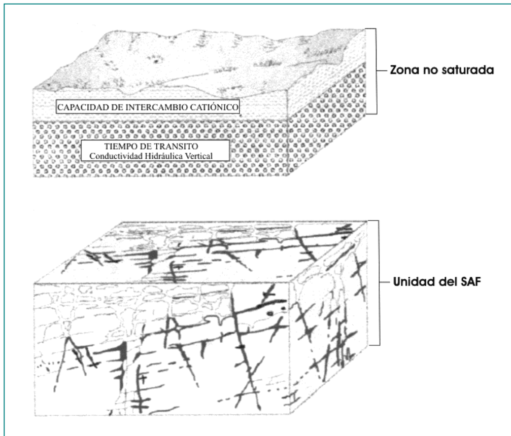
Figura 4. Importancia de la zona no saturada. Esquema
