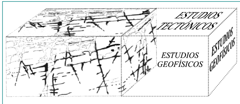
Figura 1. Geometría del SAF – Estudios directos e indirectos.
