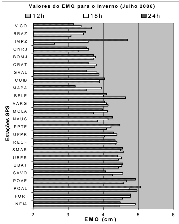
Figura 5 - Valores do EMQ para as previsões do ZTD de 12h, 18h e 24h em função das estações GPS utilizadas na avaliação para o inverno (julho de 2006).
