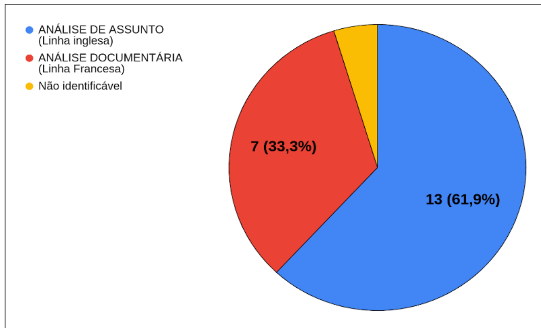
Figura 5. Correntes teóricas
