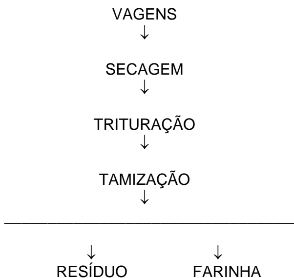
FIGURA 1 - FLUXOGRAMA DA PRODUÇÃO DA FARINHA DE ALGAROBA
