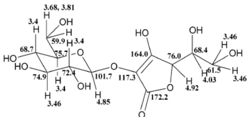
FIGURA 2 – Estrutura molecular do Ácido Ascórbico 2-O-β-Glucopiranosílico. FONTE: TOYODA-ONO et al. (2014).
